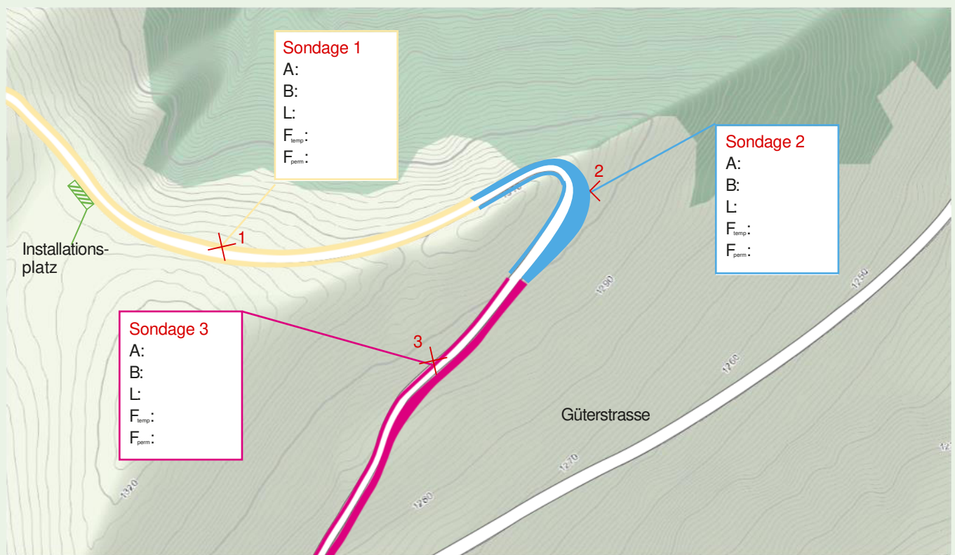
Abb. 2: Beispiel Übersichtsplan
