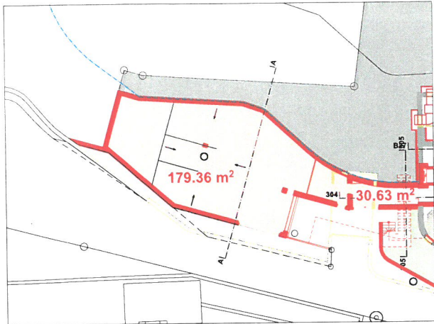
-1. UNTERGESCHOSS 1:500
